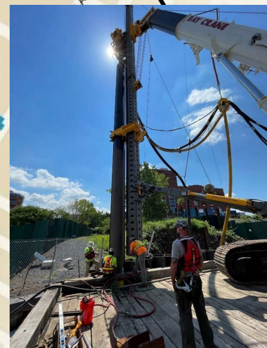
Instalación de muro de contención de pilotes tubulares en la antigua dársena de maniobras de 1st Street
